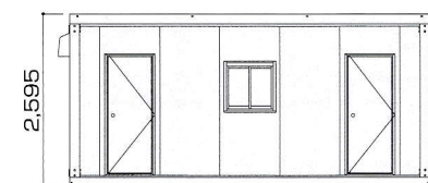
■ 立面図
