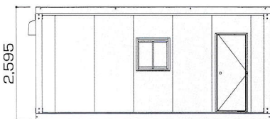
■ 立面図
