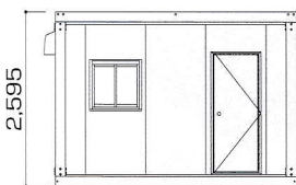
■ 立面図
