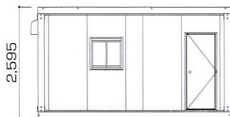
■ 立面図
